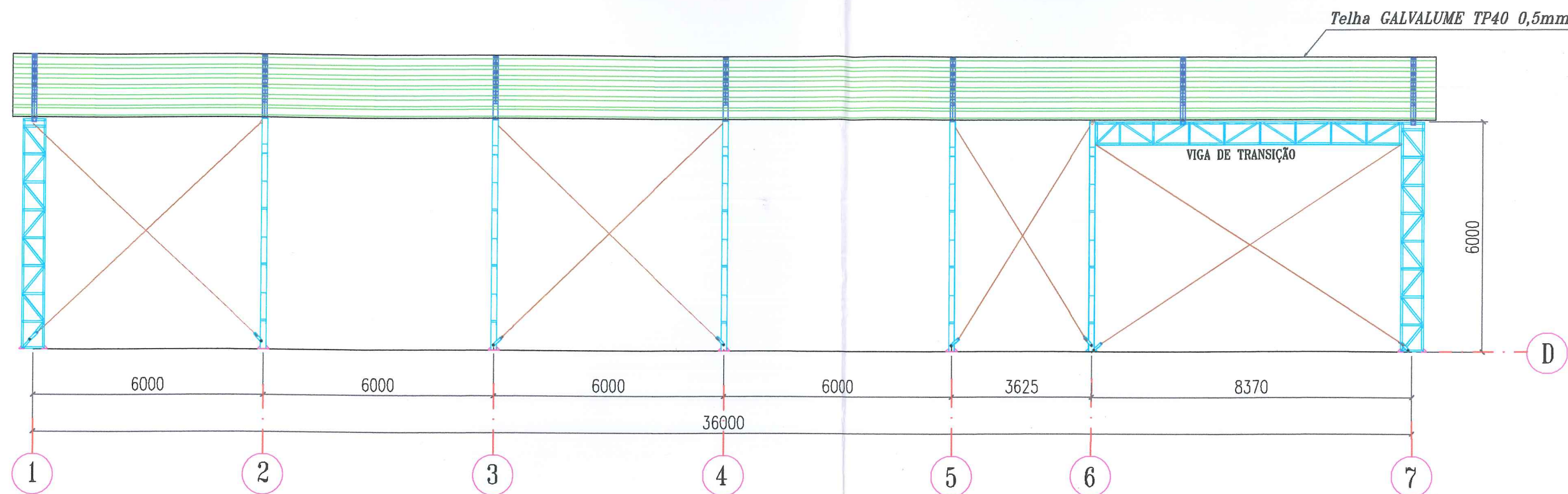
CORTE LATERAL EIXO D ESC.: 1/110
