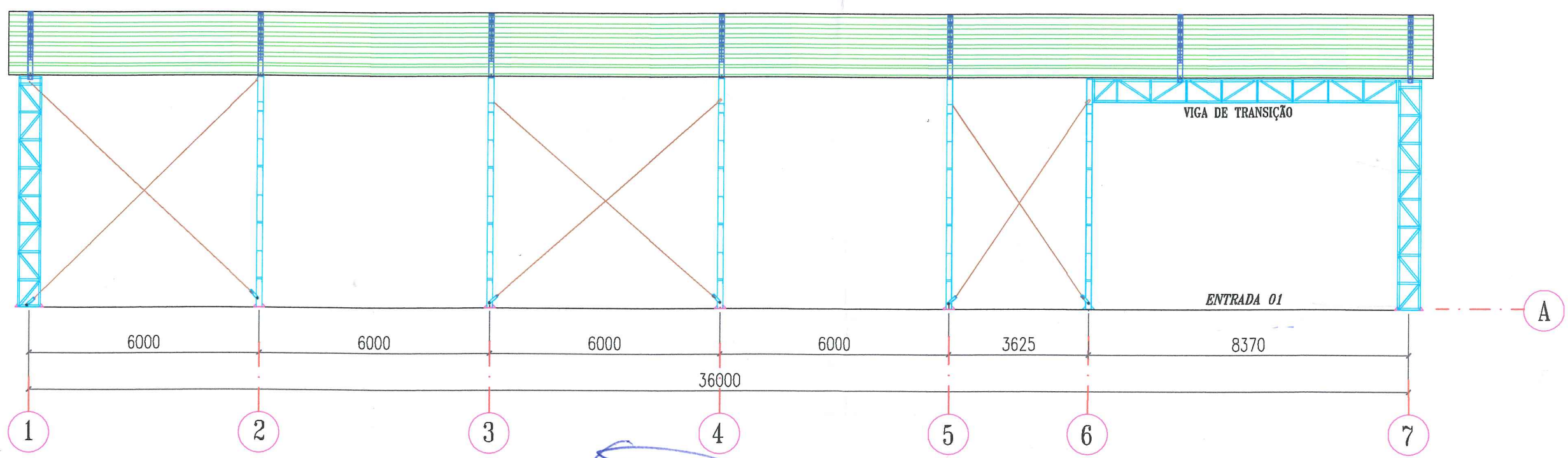
CORTE LATERAL EIXO A ESC.: 1/110
